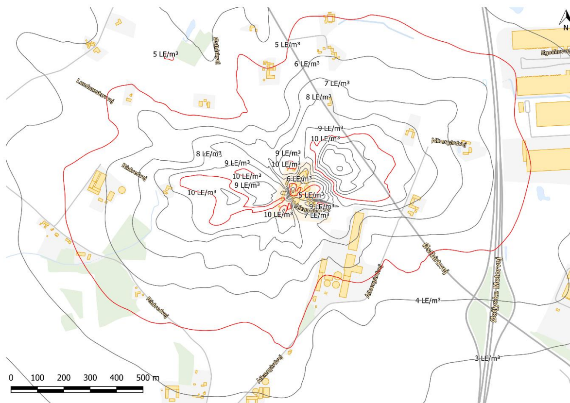
Figur 4-23: Lugtdybelsekort for lugtemissioner efter udvidelse af anlægget. Kortet illustrerer biogasanlæggets lugtbidrag ved hjælp af isolinjer med en opløsning på 1 \text{ LE/m}^3 . Det illustrerede lugtbidraget er 99 %-fraktilen fra biogasanlæggets lugtkilder, simuleret over 10 år.
