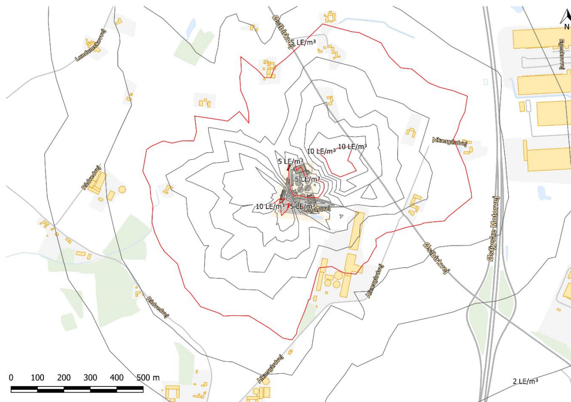
Figur 4-21: Lugtudbredelseskort for lugtemissioner før udvidelse af anlægget. Kortet illustrerer biogasanlæggets lugtbidrag ved hjælp af isolinjer med en opløsning på 1 LE/m 3 . Det illustrerede lugtbidrag er 99 %-fraktionen fra biogasanlæggets lugtkilder, simuleret over 10 år.
